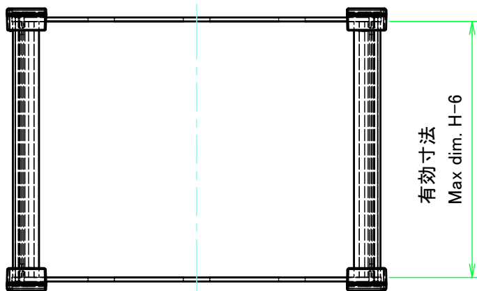
Wパネル1 / W Panel 1
