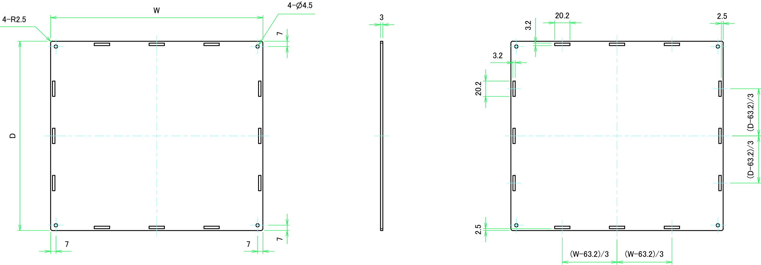
上カバー表面 / Top cover Frontside
