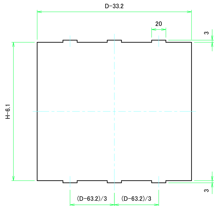
Dパネル1表面 / D Panel 1 Frontside
