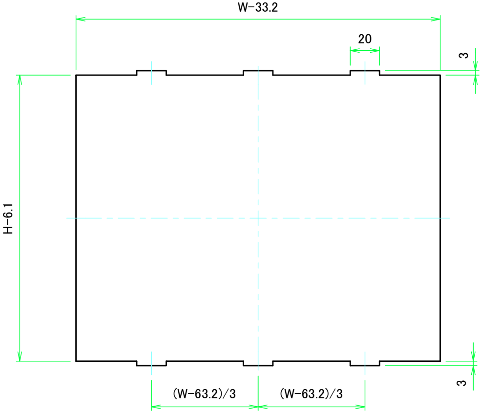
Wパネル1表面 / W Panel 1 Frontside
